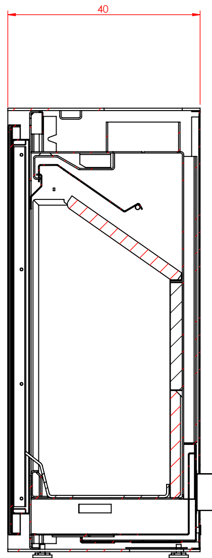
SECCIÓN G-G ESCALA 1 : 8
